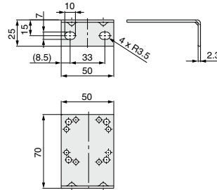
L-bracket
