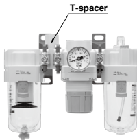
T-spacer
