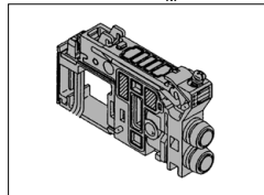
EXH block base assembly VVQ1000-19A- F□ C 3 , C 4 P□ C 6 , N 5 L□ N 7 , N 8
